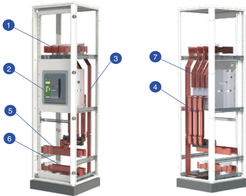
Расположение узлов схемы в конструкции шкафа ввода
