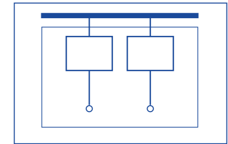
Вид внутреннего разделения 2б: выводы отделены от сборных шин
