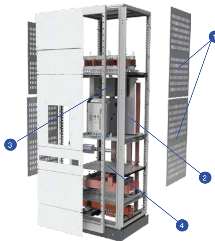
Элементы разделения функциональных блоков FBV, FBH
